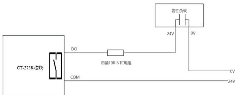
图 2 感性负载接线图
