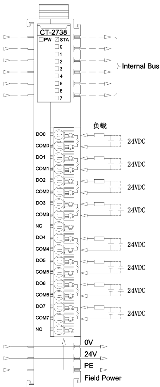
图 1 阻性负载接线图
