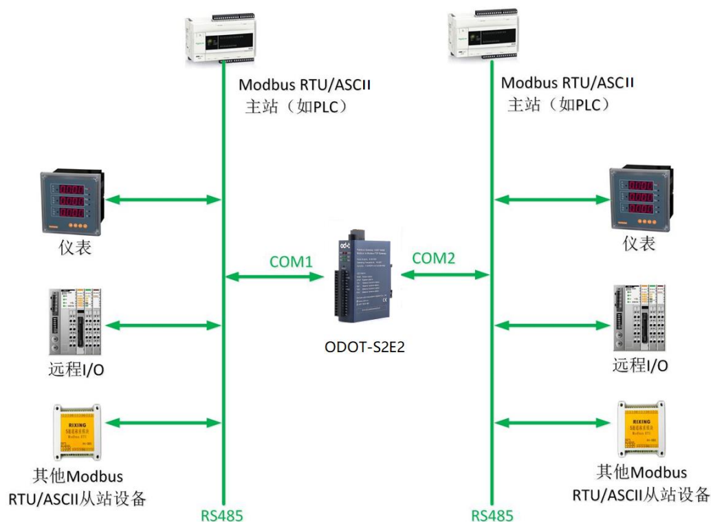
图 3.23 系统拓扑图
