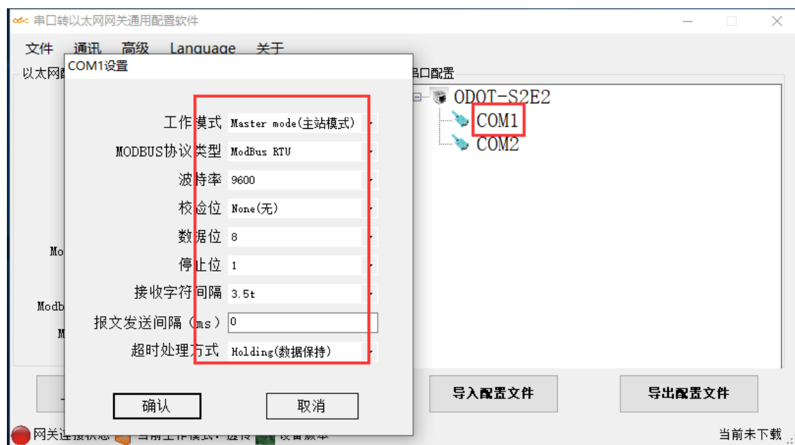
图 3.4 设置串口属性
