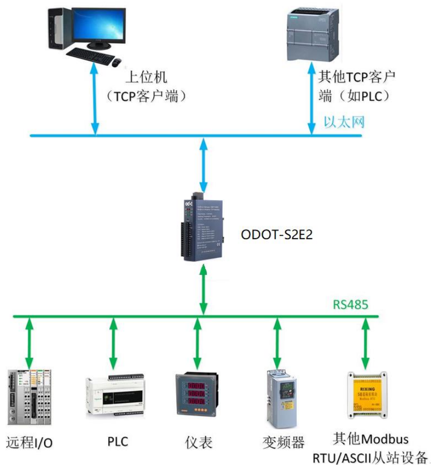
图 3.1 系统拓扑图
