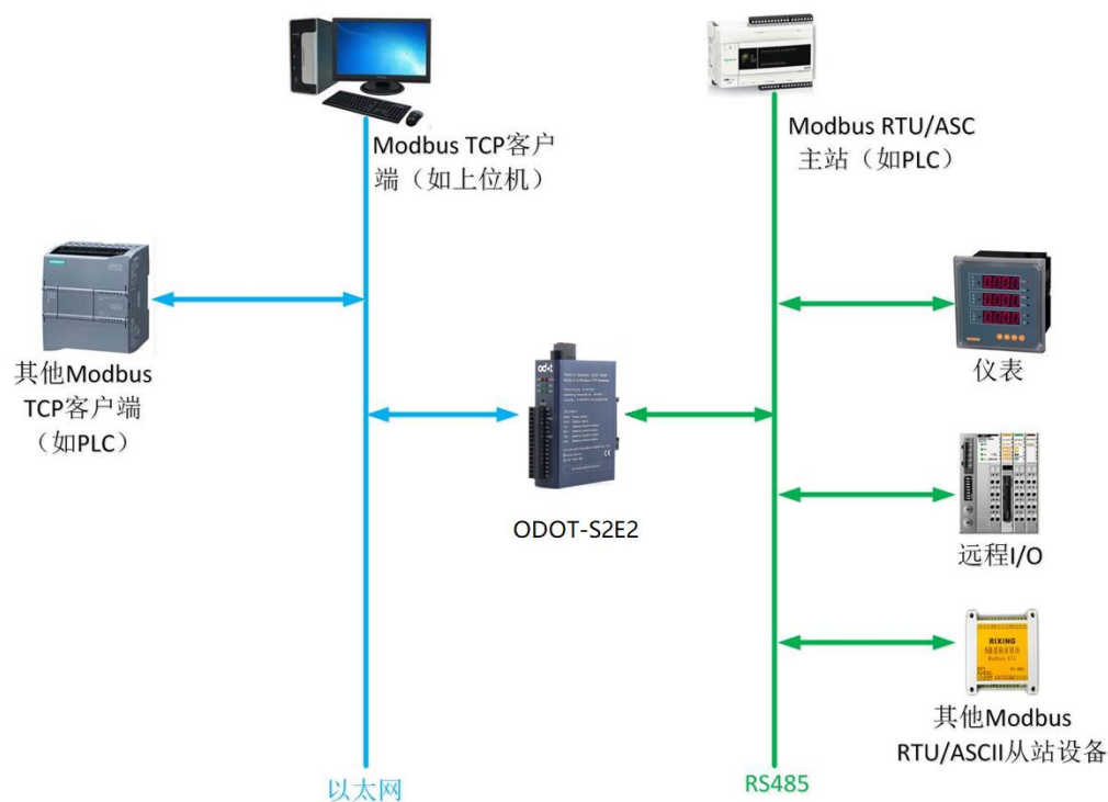
图 3.16 系统拓扑图
